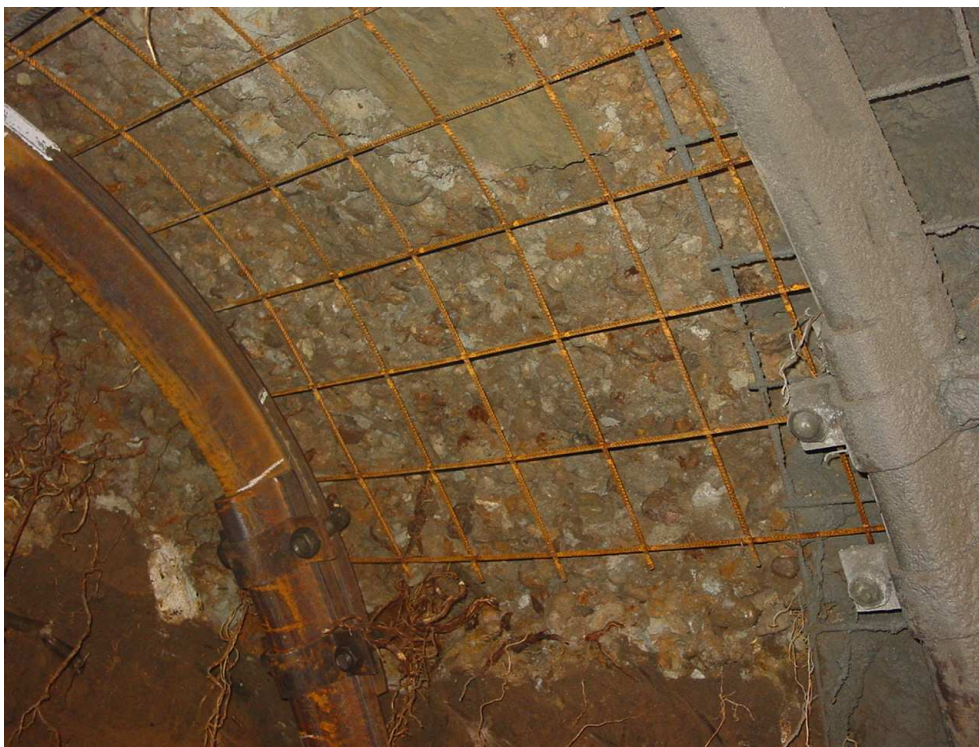
Ostění při ražbě klasickou důlní technologií
