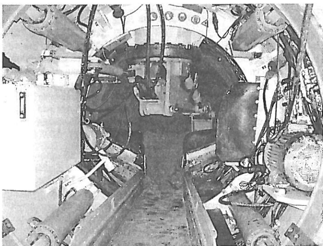
Pohled na mechanizovaný razicí štít (štola B).
