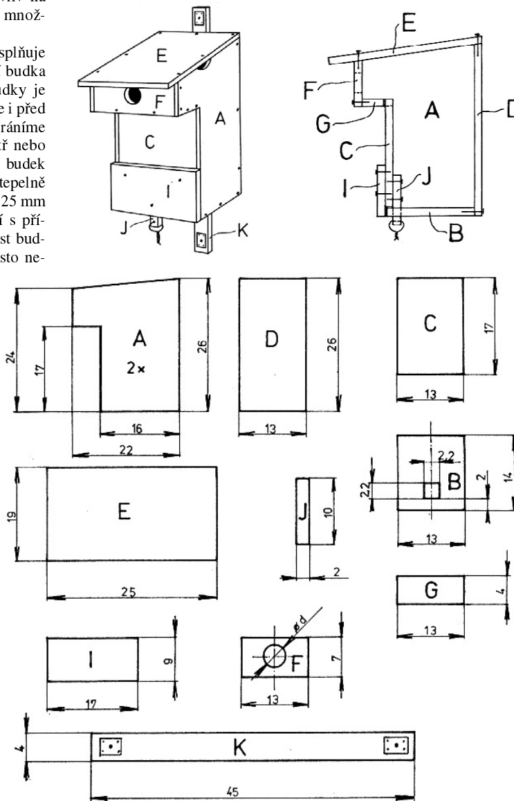
Rozměry jsou v cm. Jako materiál použijte prkna 2 cm silná, lišta K by měla být z tvrdého dřeva.
