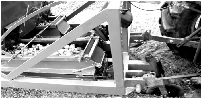
Strojová výsadba cibulovin.
